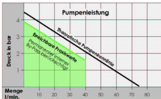
Pumpendiagramm
