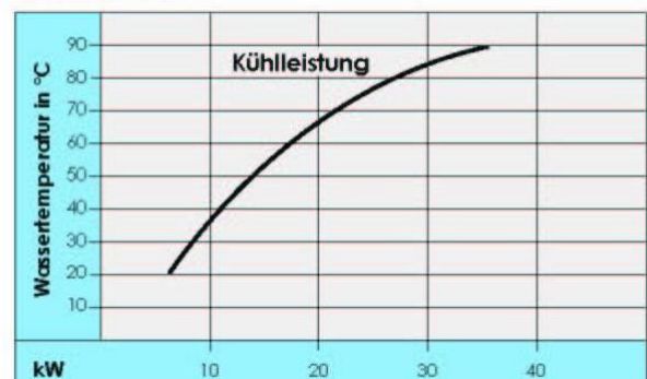
Kühlleistungsdiagramm
